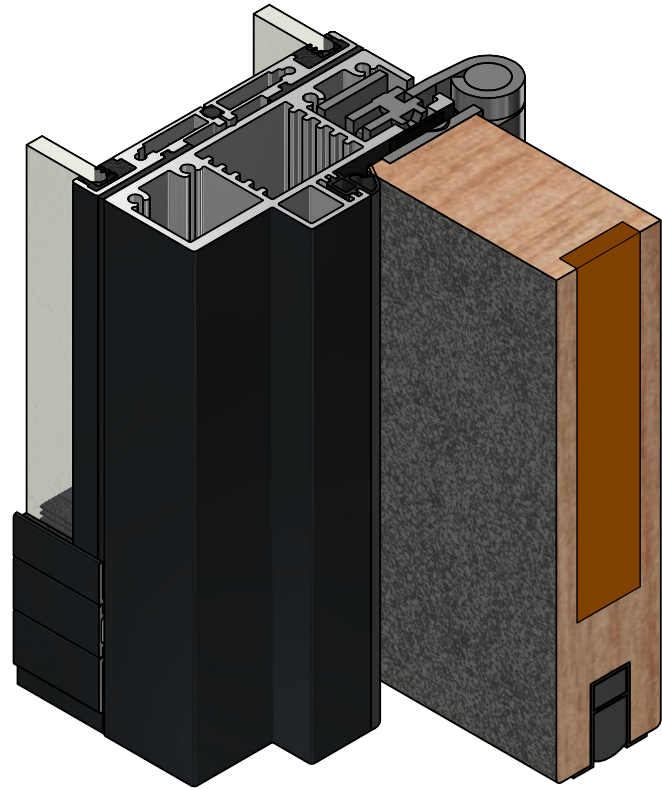
VIEW1 ( 1 : 1 )
